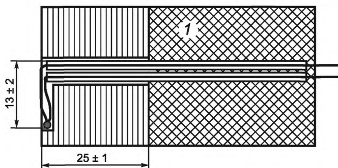
Рисунок 6 — Расположение термоэлемента в стенках испытательного угла
