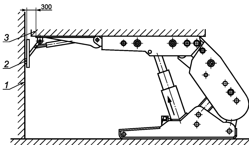
Рисунок И.1 — Схема нагружения механизма удержания забоя
