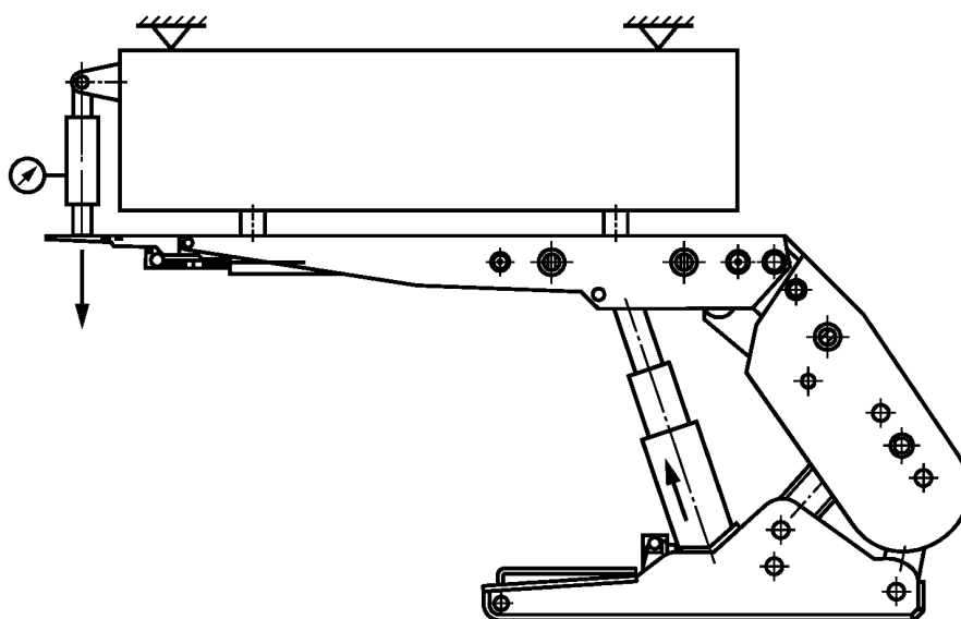
Рисунок В.4 — Схема нагружения для определения сопротивления на конце составной гидropоджимной консоли перекрытия
