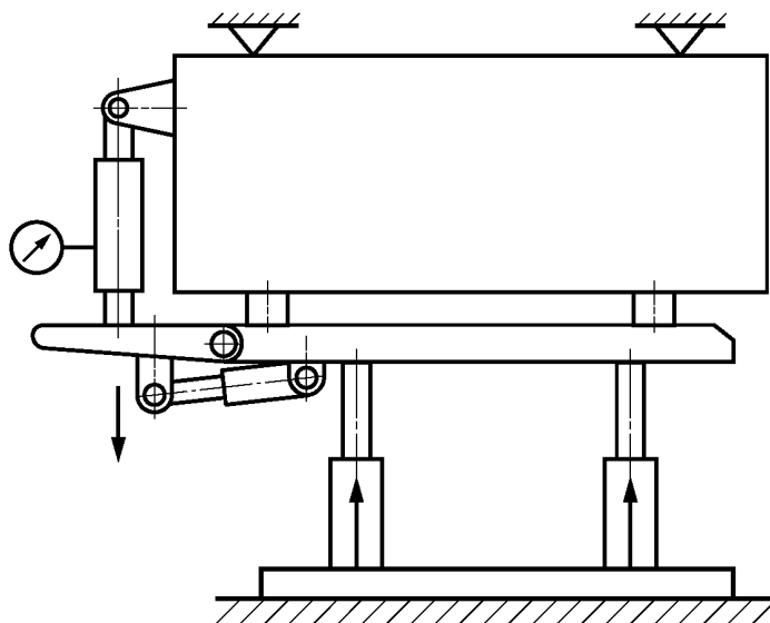
Рисунок В.3 — Схема нагружения для определения сопротивления на конце гидropоджимной консоли (козырька) перекрытия
