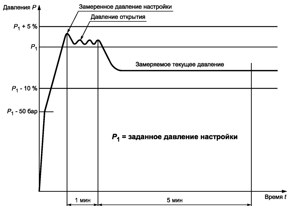
Рисунок А.2 — Пример характерного протекания процесса «давление/время» для предохранительного клапана
