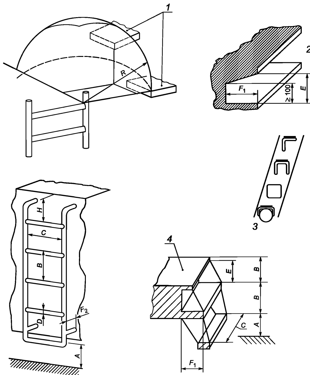
Рисунок А.2 — Ступени и лестницы погрузочных кранов
