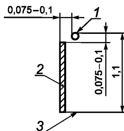
1 — поручень; 2 — боковое ограждение; 3 — пол (настил) кабины (люльки)
