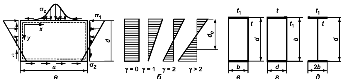
а — общий случай нагружения пластины; б — эпюры распределения нормальных напряжений \sigma ; в, г, д — обозначения расчетных размеров пластин для расчета стенки корчатой балки, пояса корчатой балки и стенки двутавровой балки.
