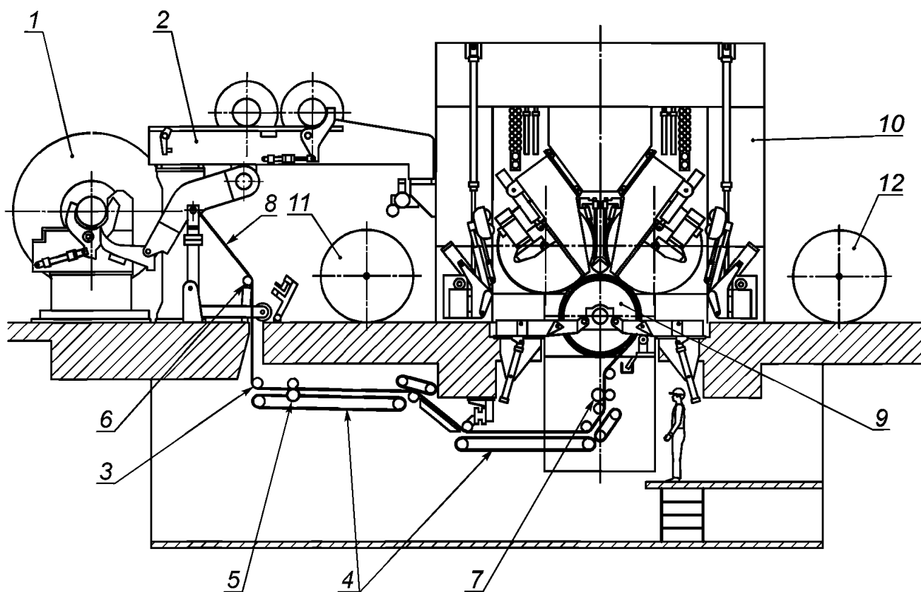
Рисунок А.9 — Принцип построения продольно-резательного станка с накопителями машинных рулонов и тамбурных валов
