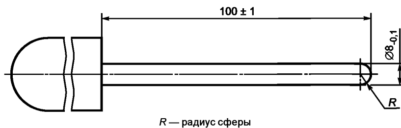
Рисунок Г.1 — Стержень-палец А (малый)
