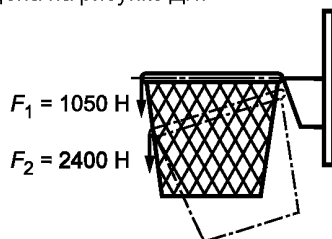
Рисунок Д.1 — Схема приложения нагрузки к кольцу с амортизатором
