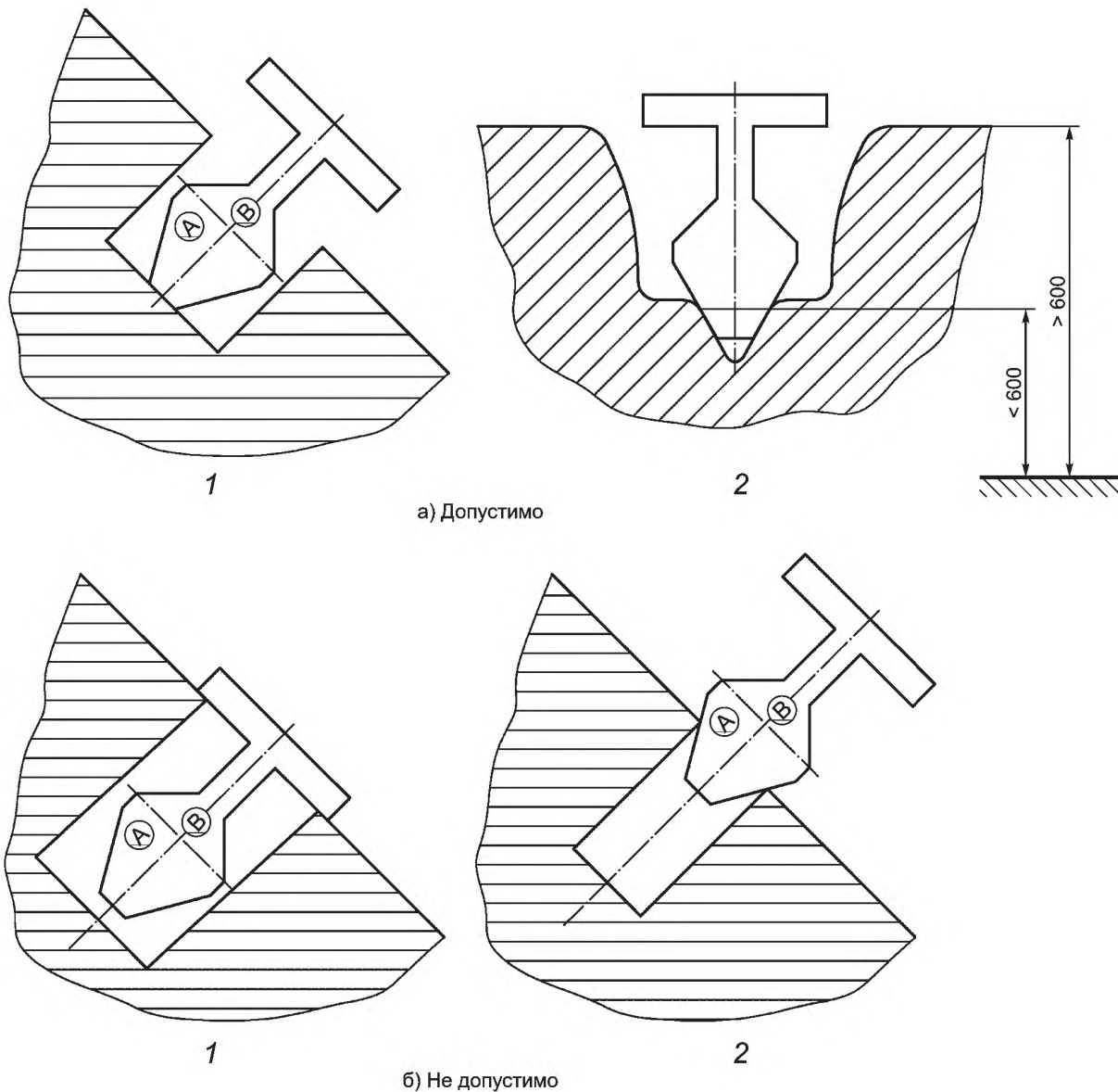
Рисунок Г.10 — Примеры размещения зоны А шаблона при испытаниях зазоров, вариант 1
