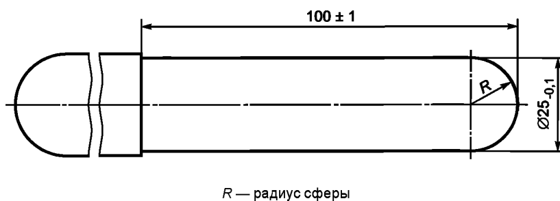
Рисунок Г.2 — Стержень-палец Б (большой)
