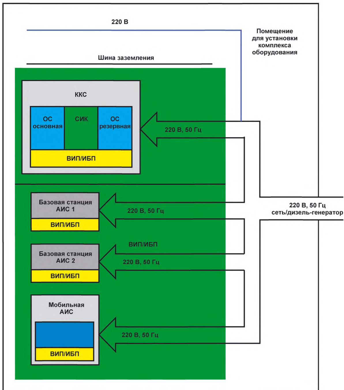
Рисунок 2 — Схема электропитания комплекса оборудования «ККС — БС — АИС» и «АИС транспондера»
