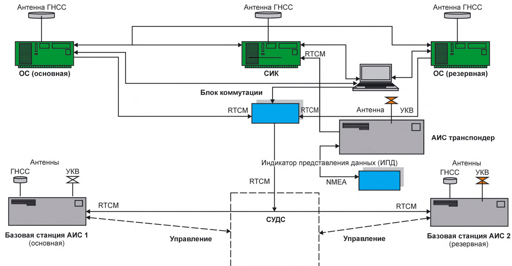
Рисунок 1 — Функциональная схема соединения аппаратуры комплекса оборудования «ККС — БС АИС — АИС транспондер»
