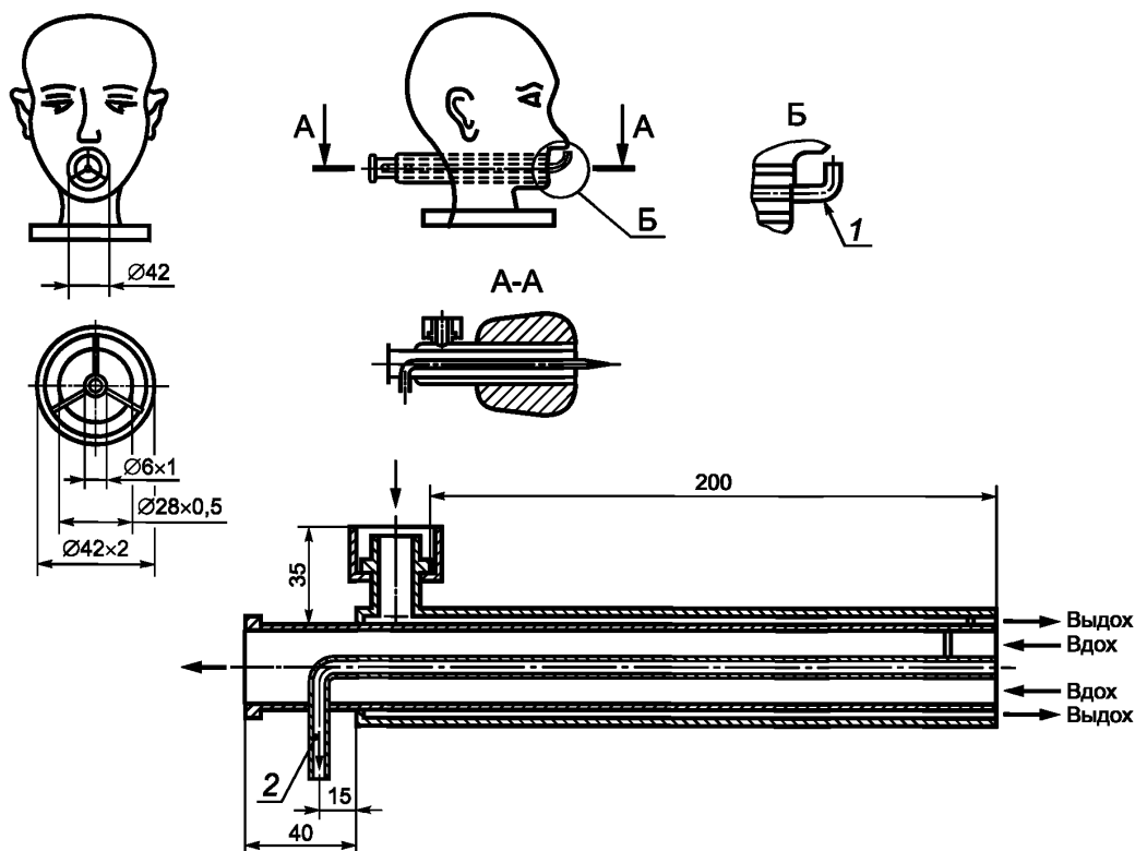
1 — втулка для измерения сопротивления воздушному потоку; 2 — измерения \text{CO}_2
