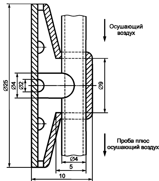
Рисунок 5 — Пробоотборник
