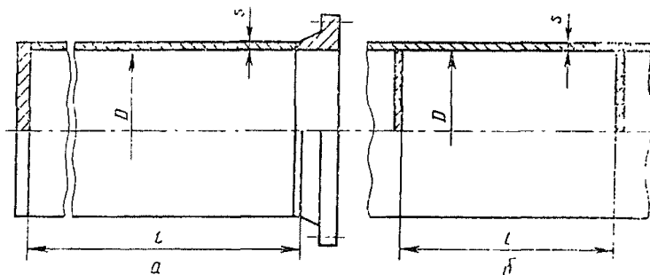
а—обечайка с фланцем или с плоским днищем, б—обечайка с жесткими перегородками
