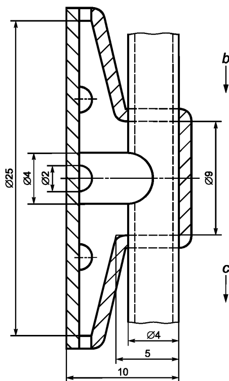
а — прозрачный материал (например, ПВХ); b — осушающий воздух; c — проба с осушающим воздухом
