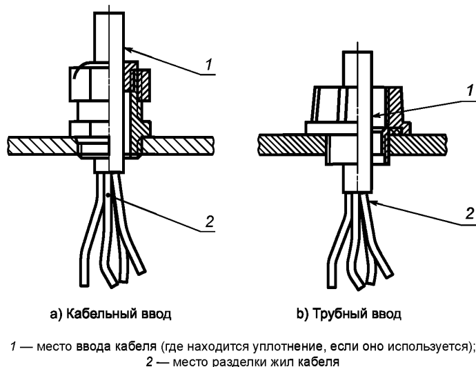
Рисунок 3 — Места ввода и разделки кабеля
