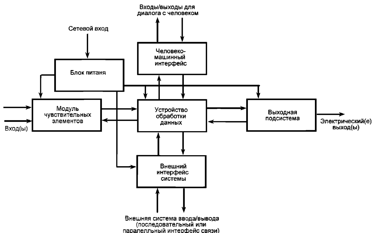
Рисунок А.1 – Модель измерительного устройства
