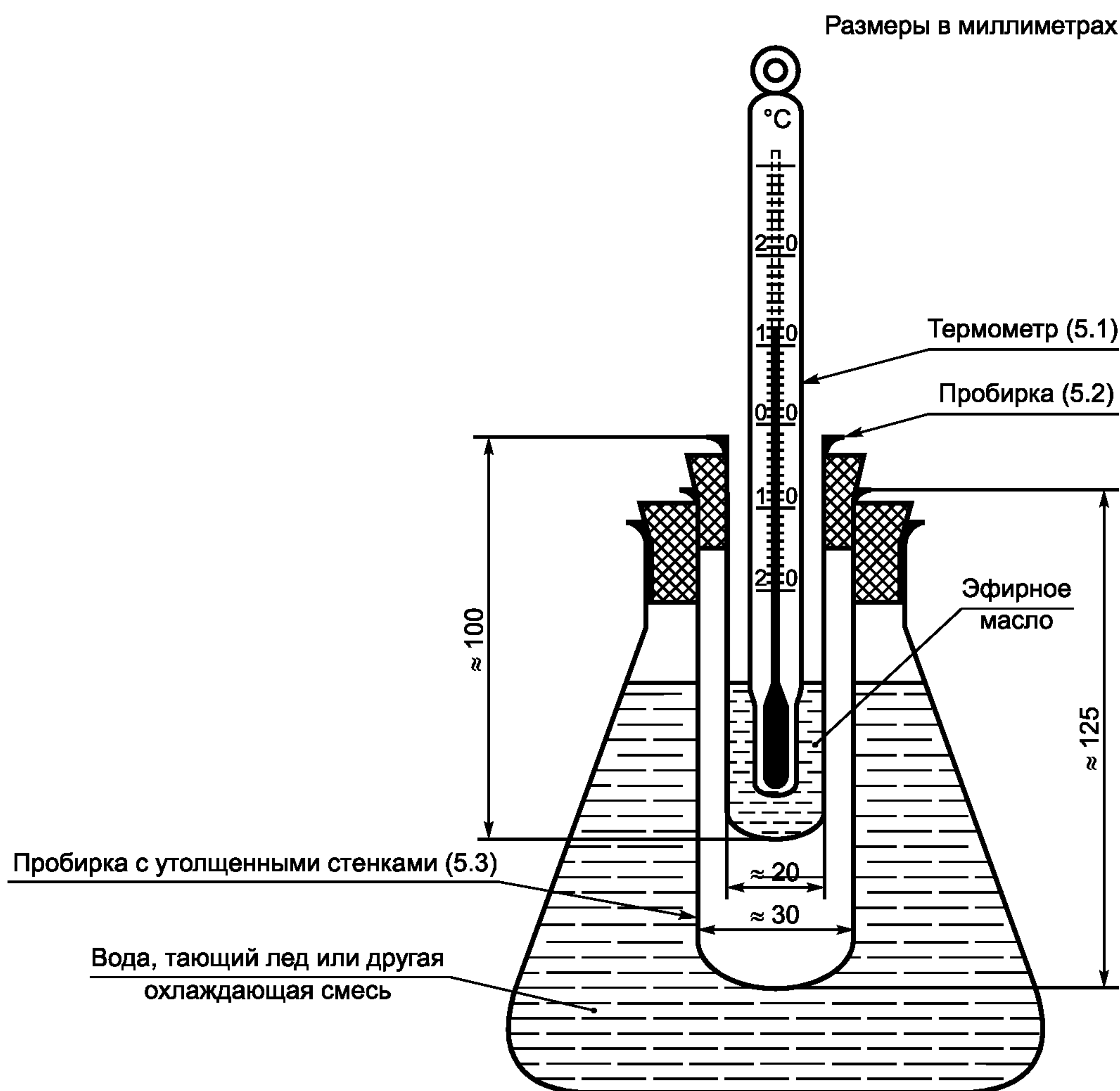
Рисунок — Подходящий прибор для определения температуры застывания
