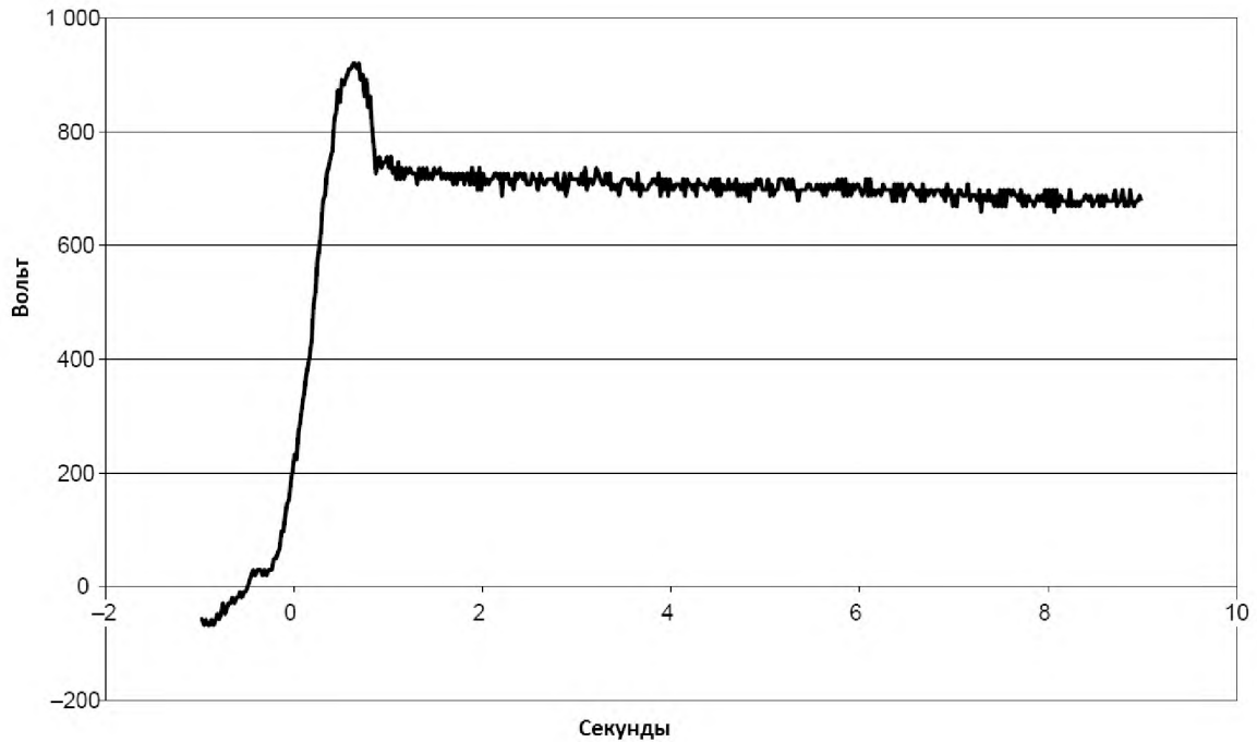
Рисунок В.2b — Электрическое напряжение тела, измеренное во время вставания с сидения поочередно каждой ногой
