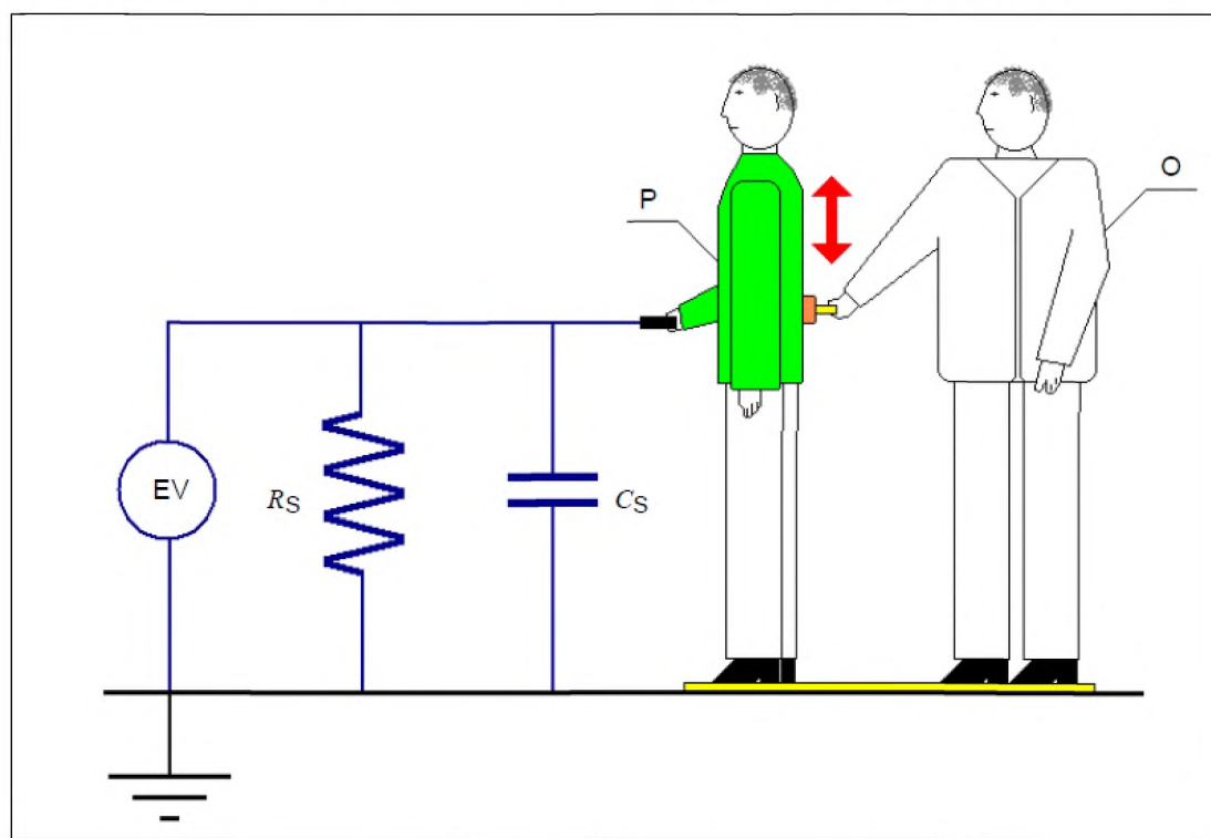
Рисунок С.8 — Схема системы для измерения уровня заряда испытуемого в результате ручного трения его одежды
