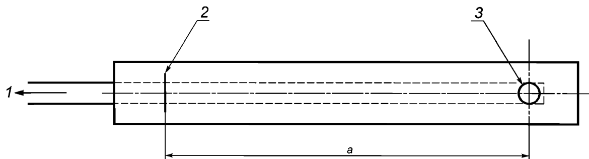
1 — натяжение; 2 — лезвие резака; 3 — направляющий стержень; а — рабочая зона
