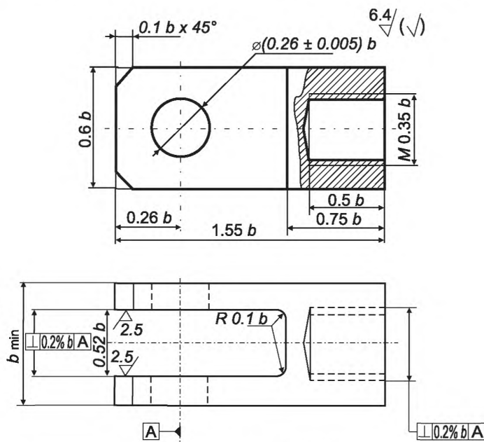
Рисунок В.3 — Рекомендуемая конструкция сери для испытания образцов на внецентренное растяжение.
