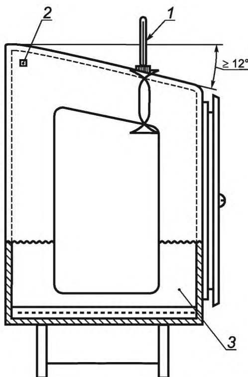
1 — термометр; 2 — клапан сброса давления; 3 — поддон наполненный водой
