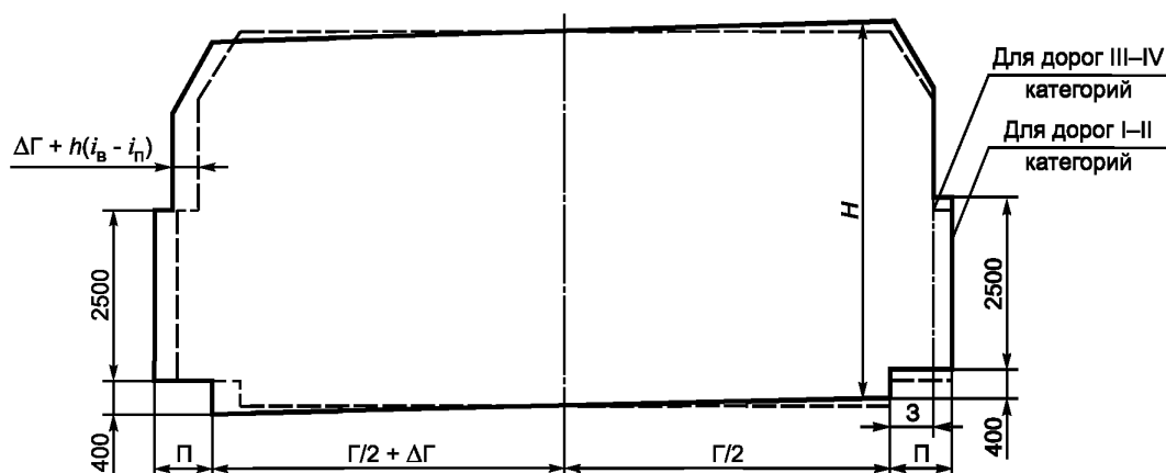
\Pi — служебный проход; З — защитная полоса; \Gamma — габарит по ширине; \Delta\Gamma — величина уширения габарита; H — габарит по высоте тоннеля; h — высота автотранспортного средства; i_B, i_{\Pi} — поперечные уклоны проезжей части на вираже и на прямой
