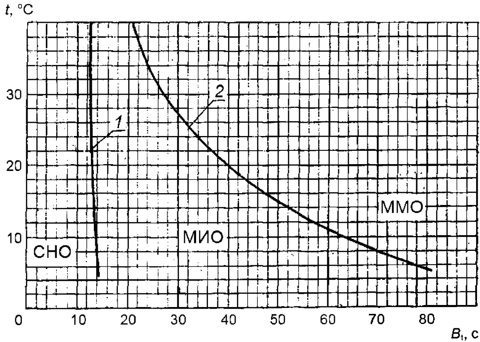
Рисунок 1 — Зависимость условной вязкости от температуры
