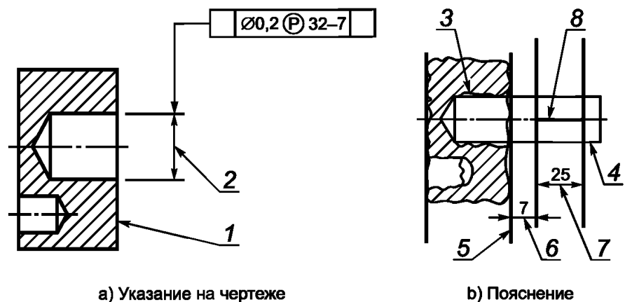
1 — опорная поверхность; 2 — указание на то, что нормируемым элементом является средний элемент (эквивалентно знаку \textcircled{A} ); 3 — реальный элемент; 4 — продолженный элемент; 5 — опорная плоскость; 6 — смещение; 7 — длина нормируемого элемента; 8 — выступающий нормируемый элемент
