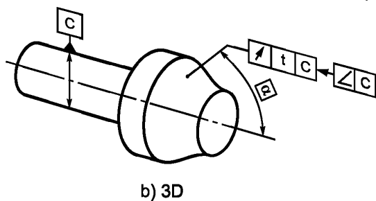
Рисунок 19 — Указание на чертеже
