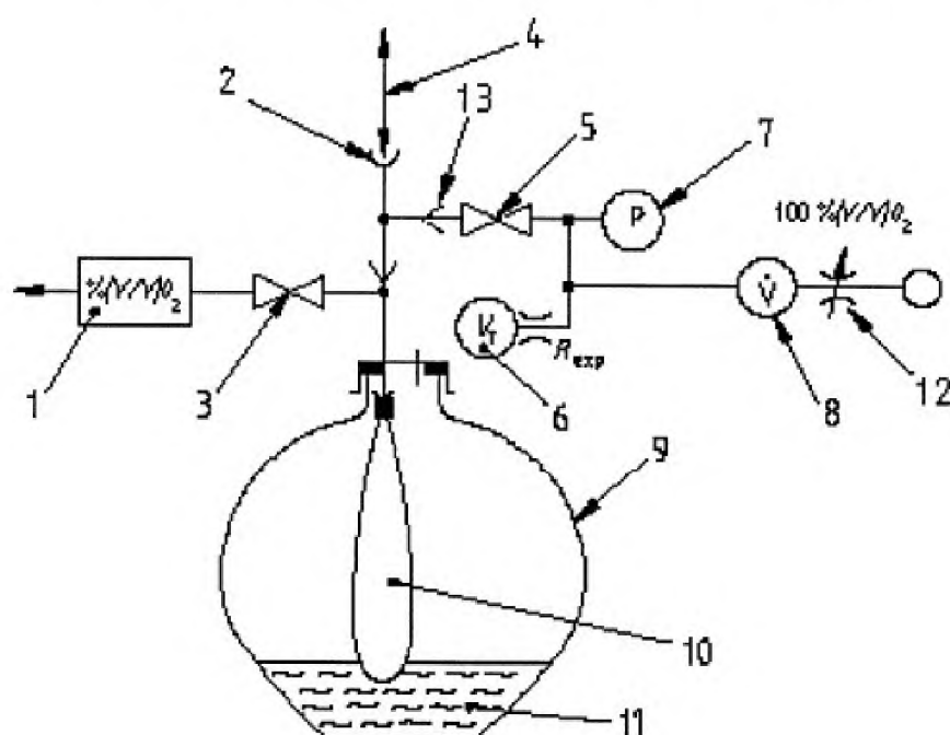
а) Испытательный коннектор для определения мертвого пространства системы V_{D,system}
