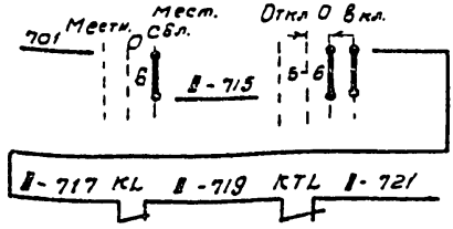
В схему сигнализации л.АЭМ-10
