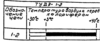
Диаграмма работы контактов датчика температуры "SK3"
