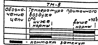
Диаграмма работы контактов датчика температуры "SK2"
