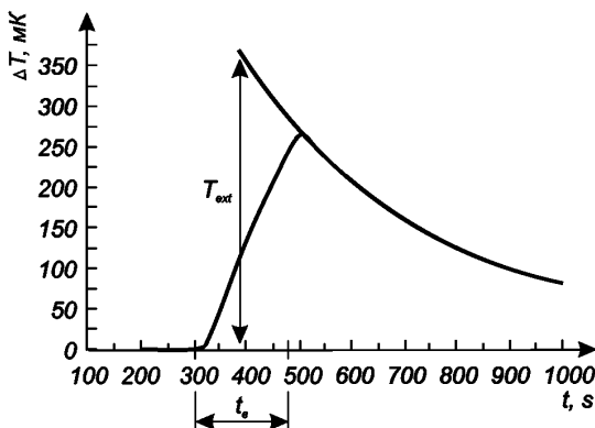
Рисунок 3 – Пример для импульсного метода оценки
