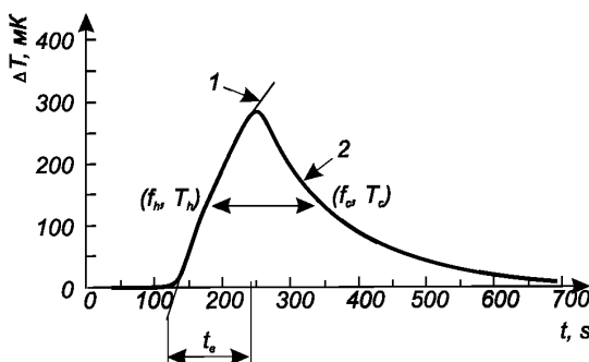
Рисунок 2 – Пример для экспоненциального метода оценки
