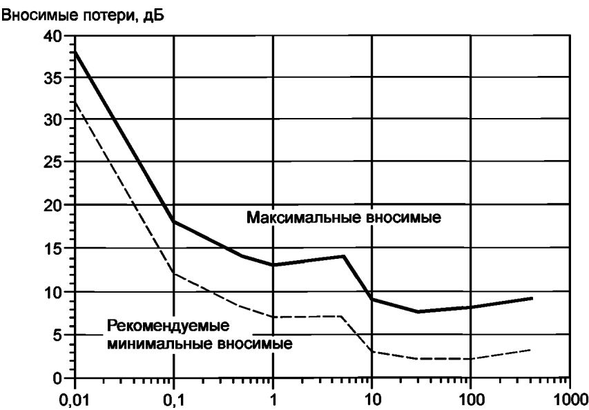
Рисунок Е.2 — Нормы вносимых потерь токового зонда
