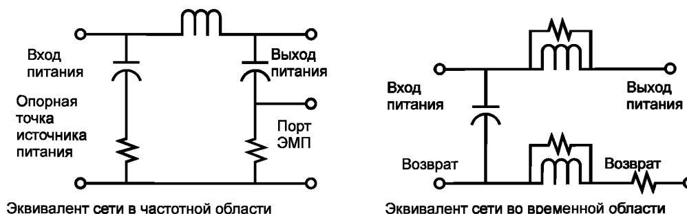
Рисунок Г.1 — Схемы эквивалентов сети
