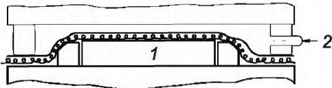
1 – уложенные слои препрега (рисунок 3); 2 – подача сжатого воздуха
