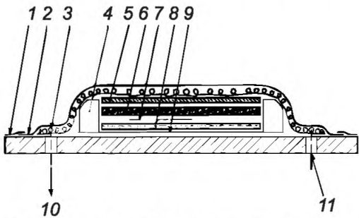
1 – уплотняющая лента; 2 – мембранное полотно; 3 – проницаемый материал; 4 – металлический брусоч; 5 – верхняя формовочная пластина; 6 – впитывающий материал; 7 – перфорированная антиадгезионная пленка; 8 – уложенные слои препрега; 9 – антиадгезионная пленка; 10 – вентиляционный канал за пределами автоклава; 11 – отверстие для подсоединения, например, температурных датчиков и/или датчиков давления
