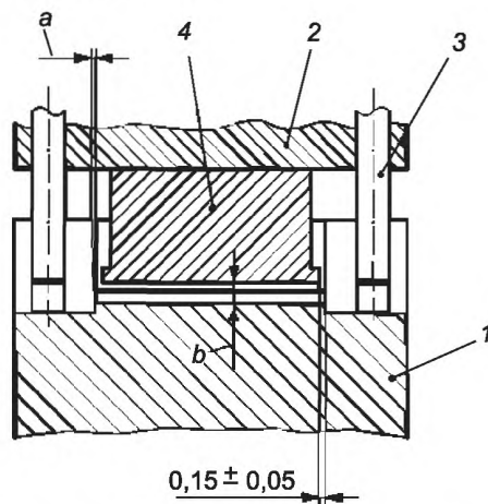
Рисунок 1 – Пресс для формования
