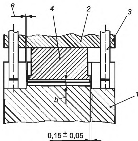
1 – основание; 2 – верхняя рама; 3 – направляющие; 4 – поршень; а – уклон по всему периметру 1°; b – режущие края по всему периметру
