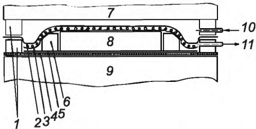
1 – металлические брусочки; 2 – мембранное полотно; 3 – проницаемый материал; 4 – опорная формовочная пластина; 5 – антиадгезионная пленка; 6 – резиновый уплотнитель; 7 – верхняя формовочная пластина; 8 – уложенные слои препрега (рисунок 3); 9 – нижняя опорная плита пресса; 10 – подача сжатого воздуха; 11 – откачивание воздуха
