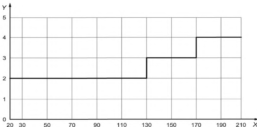
X – температура отверждения, °C; Y – допустимое отклонение температуры, °C Рисунок 5 – Примеры допустимых отклонений температуры от температуры отверждения
