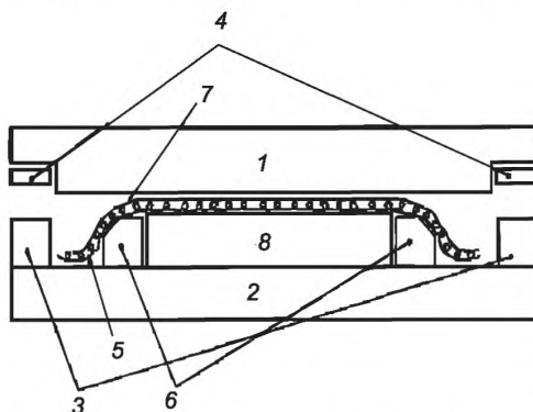
Рисунок 6 – Схема формования пластин в мембранном прессе (вакуумный метод)
