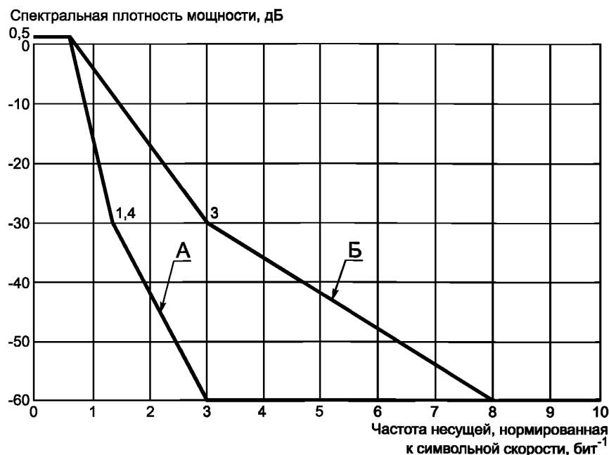
Рисунок 1 — Спектральные маски SFCG 21-2
