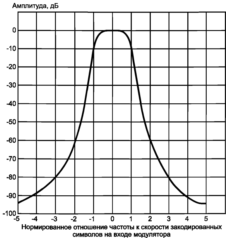
Рисунок 14 — АЧХ фильтра Бесселя 6-го порядка
