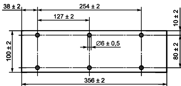
Рисунок 1 — Образец для испытаний
