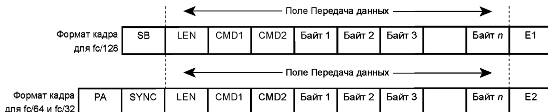
Рисунок 13 — Формат кадра передачи данных
