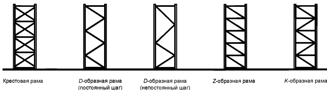
Рисунок 1 — Типовые формы рам стеллажей
