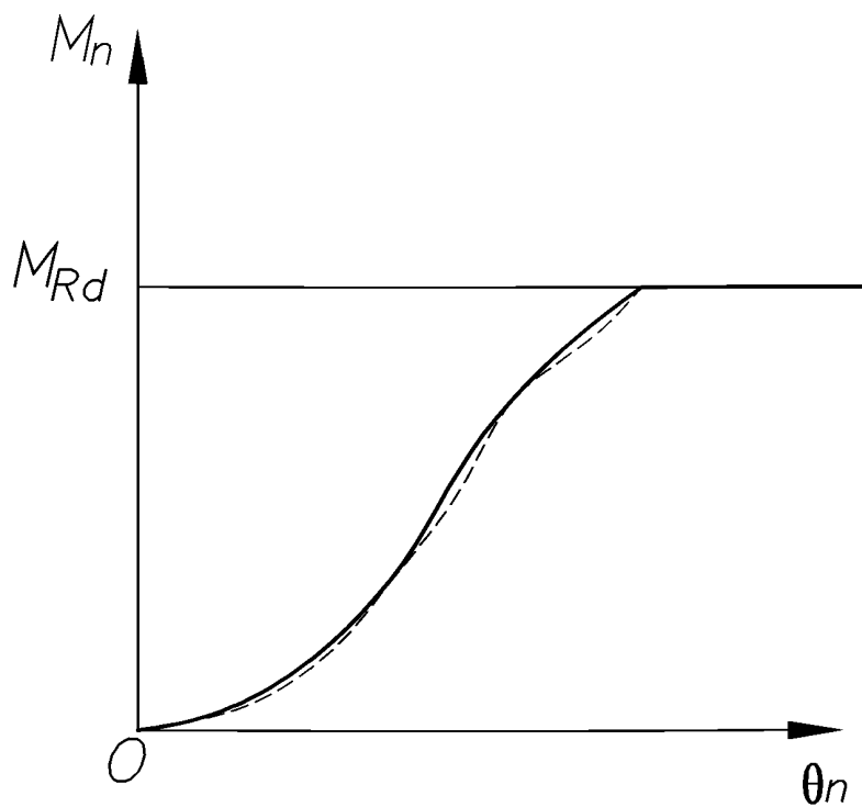
Рисунок А.8 — Типовая линеаризация средней кривой
