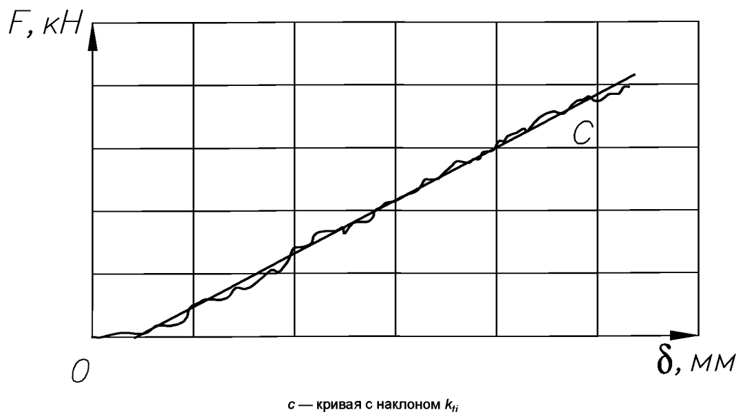
Рисунок А.14 — Кривая нагружения – деформации
