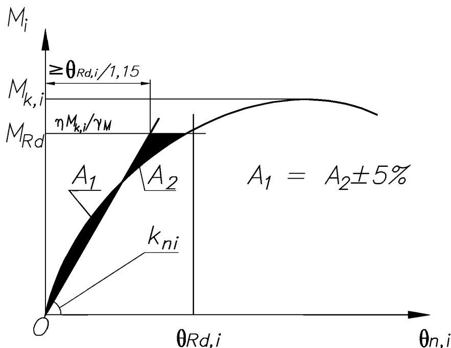
Рисунок А.6 — Обработка значений жесткости кронштейна балки
