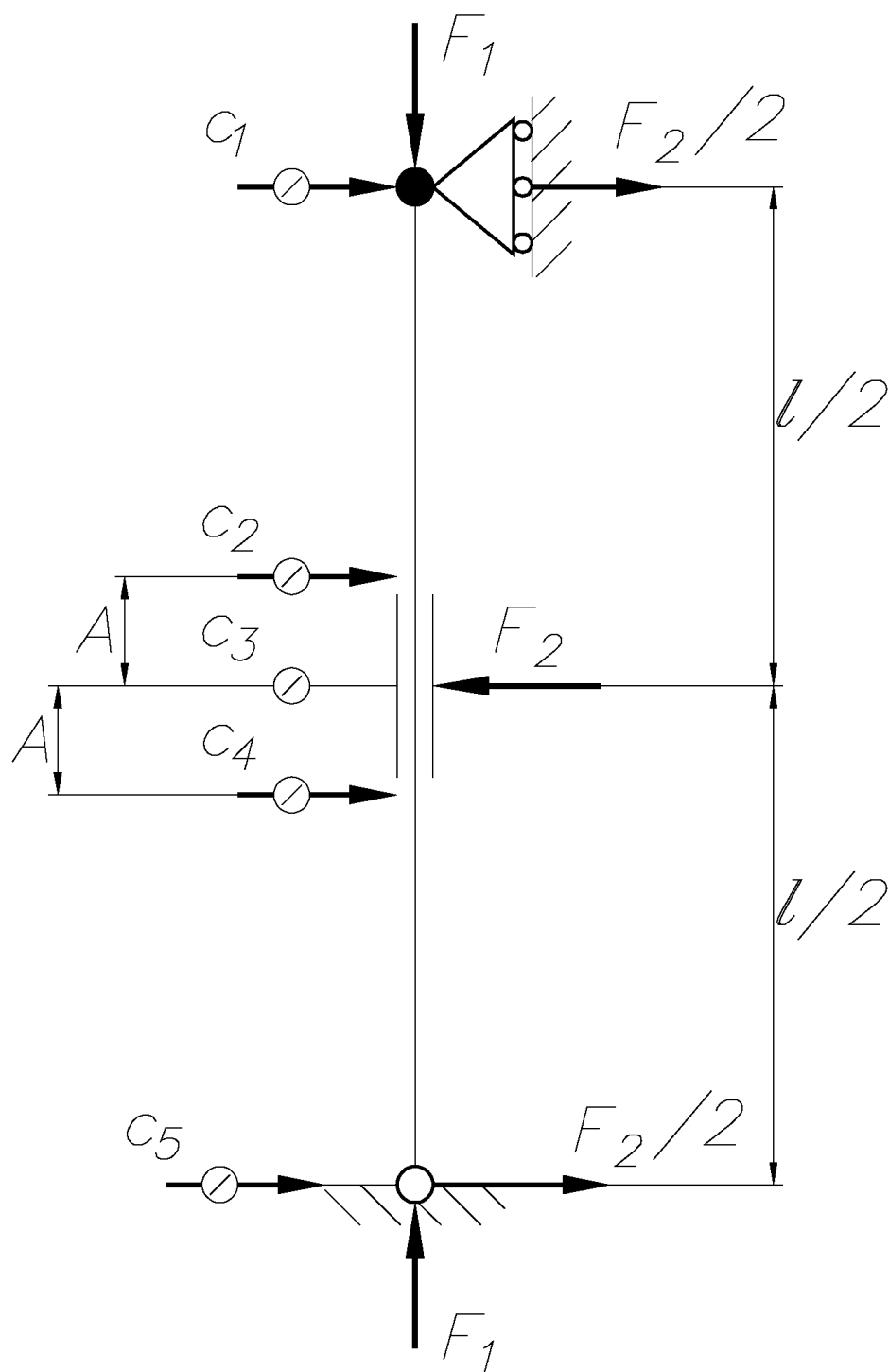
Рисунок А.17 — Порядок проведения испытаний
