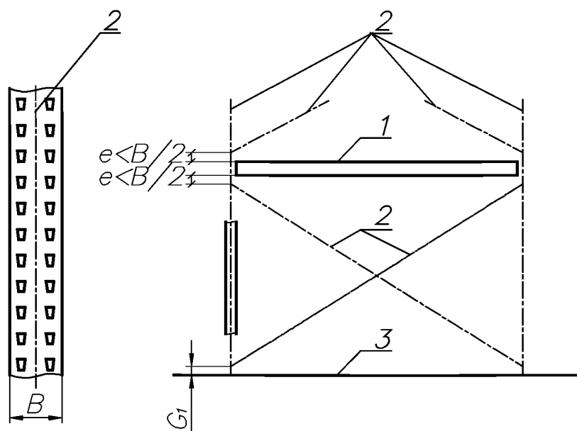
1 — балка; 2 — центральные оси элементов; 3 — пол; В — ширина стойки; е — эксцентриситет (расстояние между узлом раскоса до верхней или нижней части балки); G_1 — расстояние от пола до нижней точки узла раскоса
