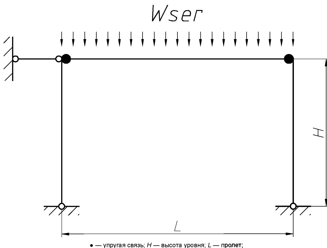
Рисунок 18 — Схема для предварительного расчета прогиба балки
