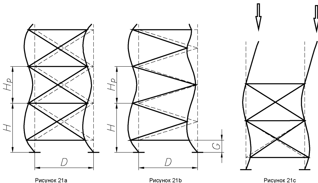
Рисунок 21 — Формы потери устойчивости рам в одной плоскости
