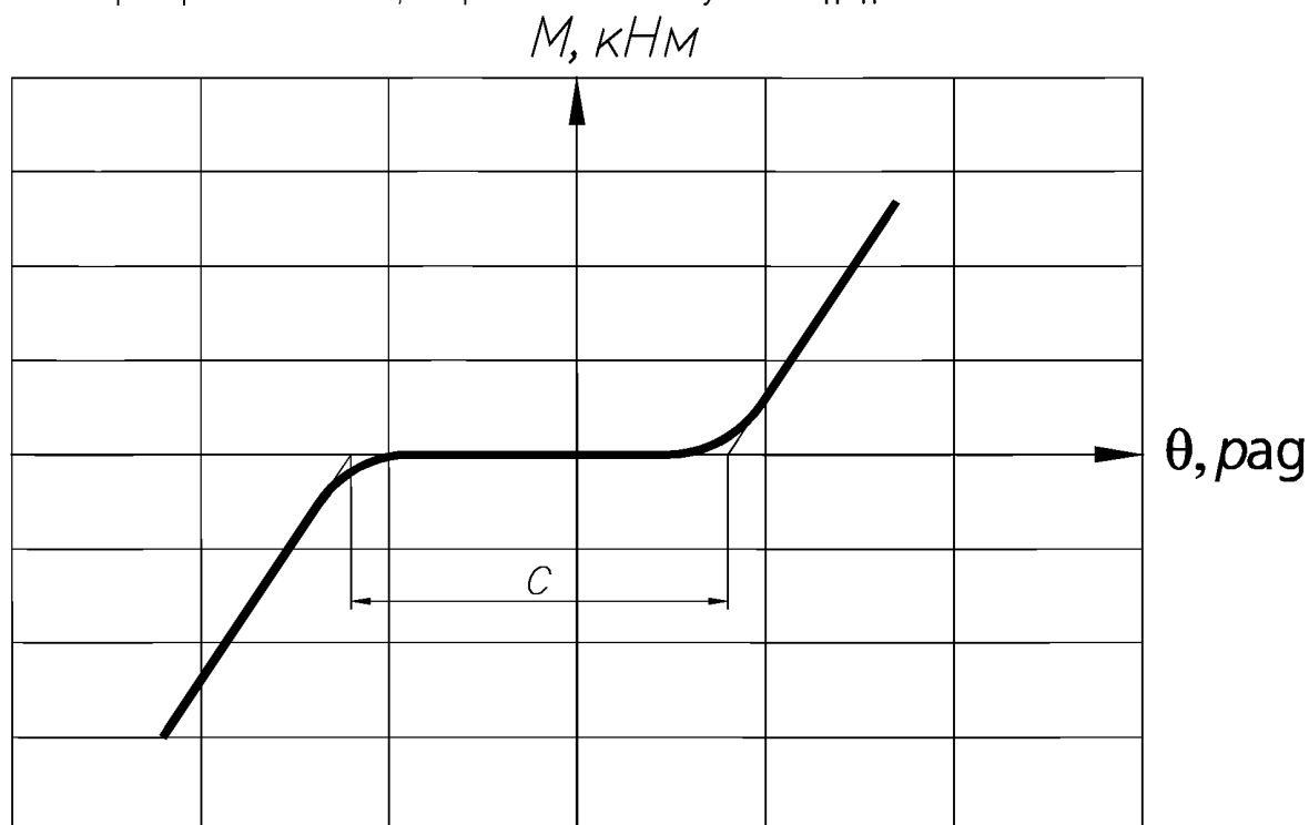
Рисунок A.9 — Характерная зависимость, получаемая в ходе испытаний.
