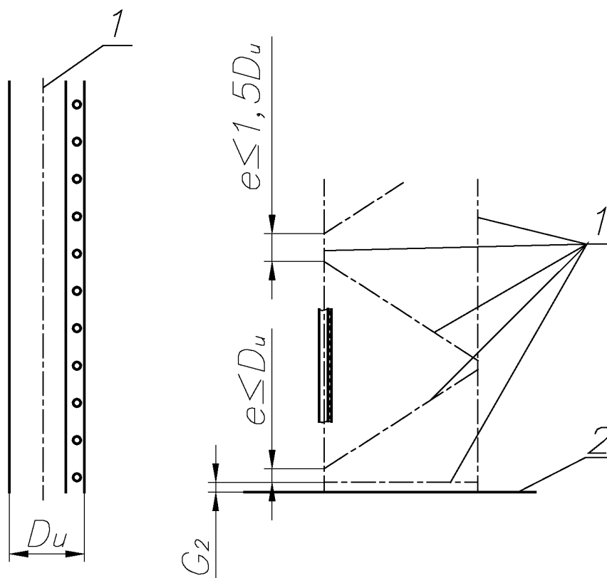
Рисунок 10b — Эксцентриситеты раскосной системы рамы
