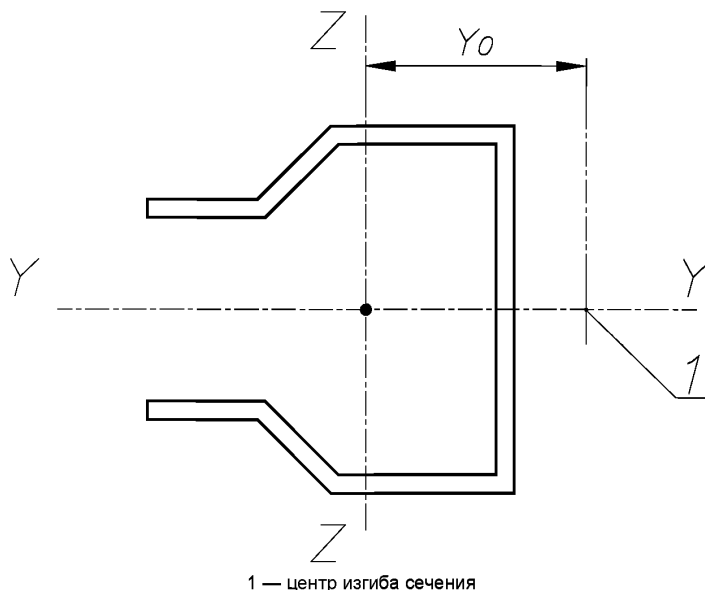
Рисунок 23 — Центр изгиба сечения
