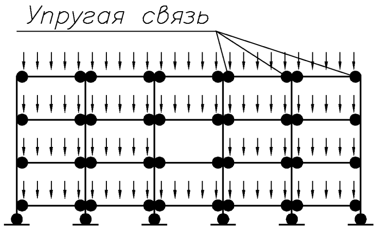
Рисунок 27 — Схемы нагружения для расчета в X-направлении
