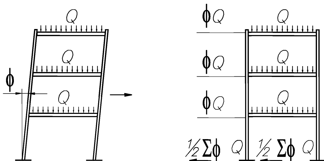
Рисунок 7 — Эквивалентные горизонтальные усилия
