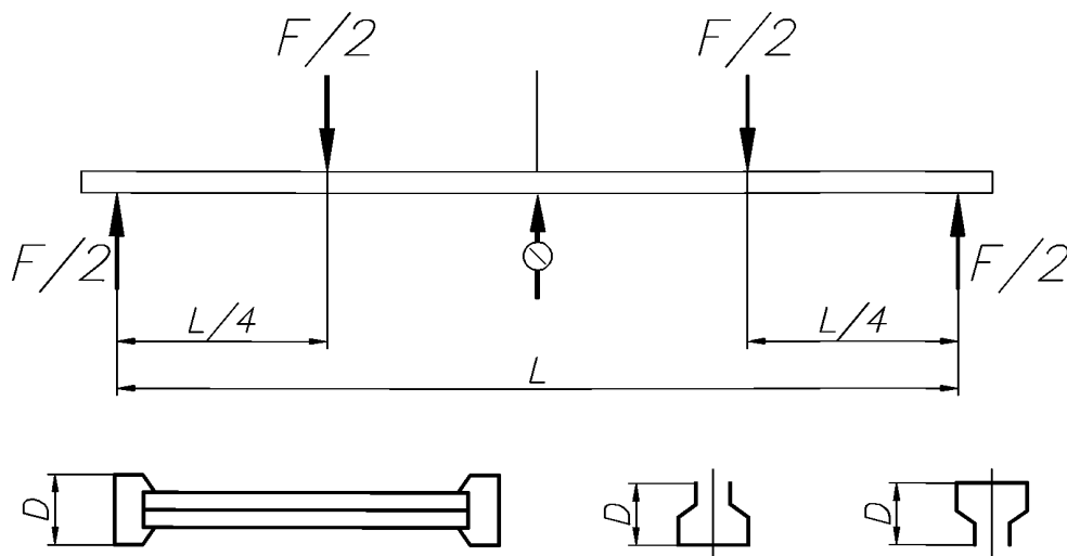
Рисунок А.15 — Порядок проведения испытаний
