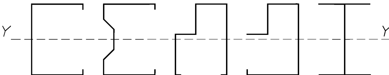
Рисунок 20 — Примеры балок, для которых вероятна потеря устойчивости плоской формы изгиба балок
