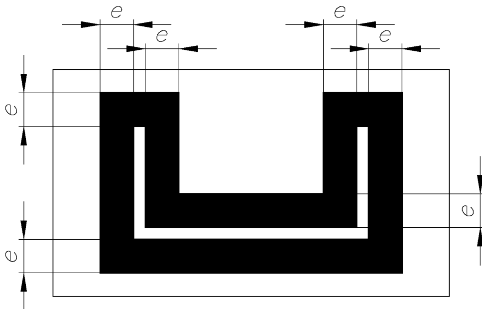
Рисунок 26 — Эффективная площадь для расчета подпятника
