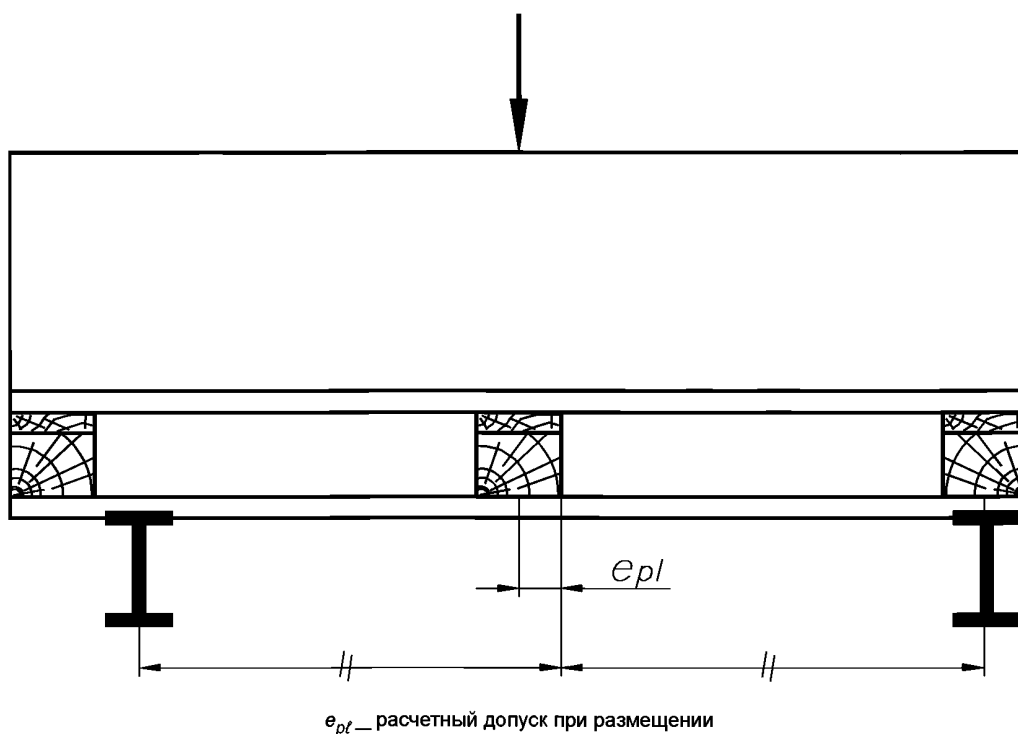
Рисунок Е.1 — Эксцентриситет нагрузки
