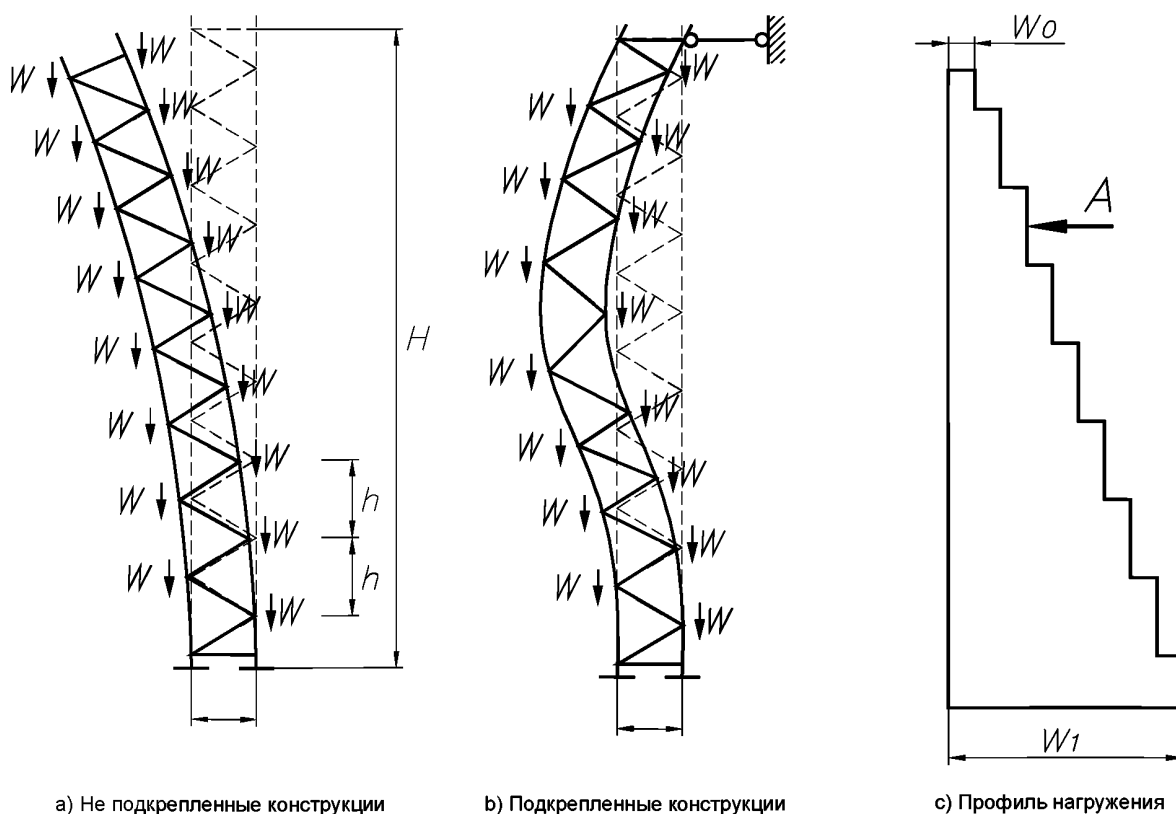
Рисунок Г.1 — Допущения для упрощенного анализа устойчивости в Y-направлении
