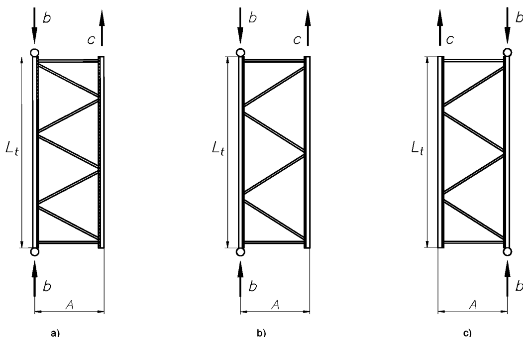
Рисунок А.3 — Порядок альтернативного проведения испытаний стоек на сжатие
