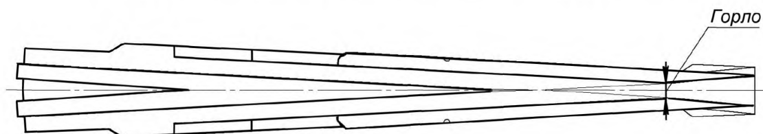
Рисунок 3.2 — Положение горла литого сердечника сборной крестовины
