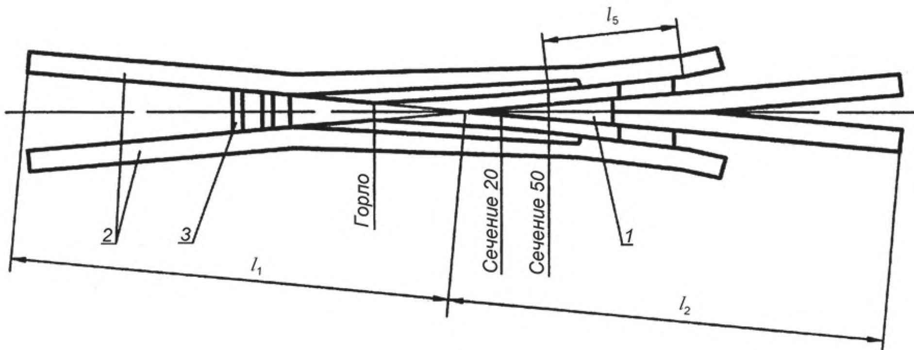
Рисунок 4.2 — Сборная крестовина без передней врезки (сочленение по косому переднему стыку) с литым сердечником и приварными рельсовыми окончаниями
