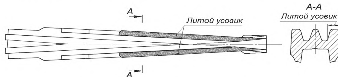
Рисунок 3.10 — Литые усовики сердечника сборной крестовины
