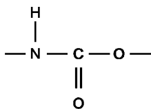
Рисунок А.1 — Уретановые группы
