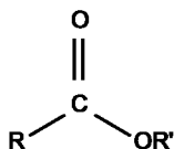
Рисунок А.2 — Эфирная связь
