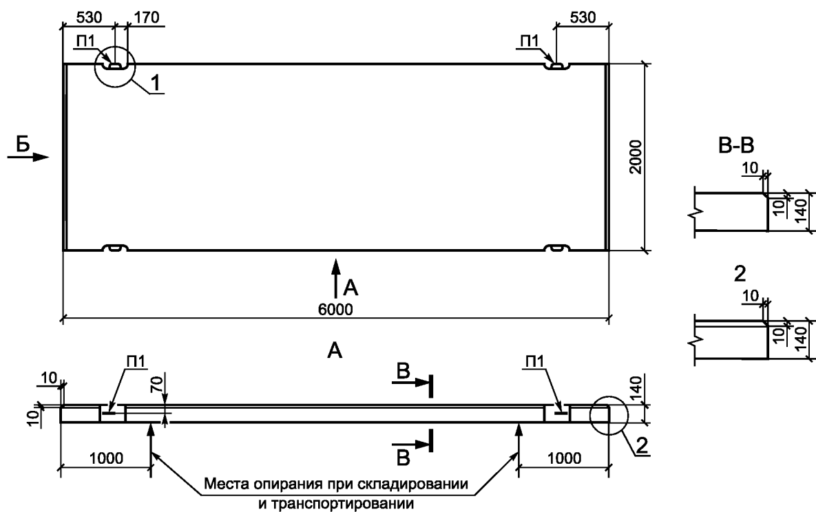
Рисунок 3 — Плита дорожная 2ПДН-14. Общий вид
