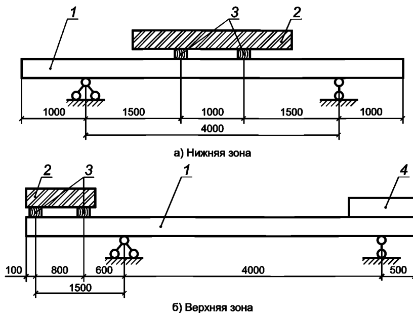
Рисунок 7 — Схемы испытания плит на трещиностойкость
