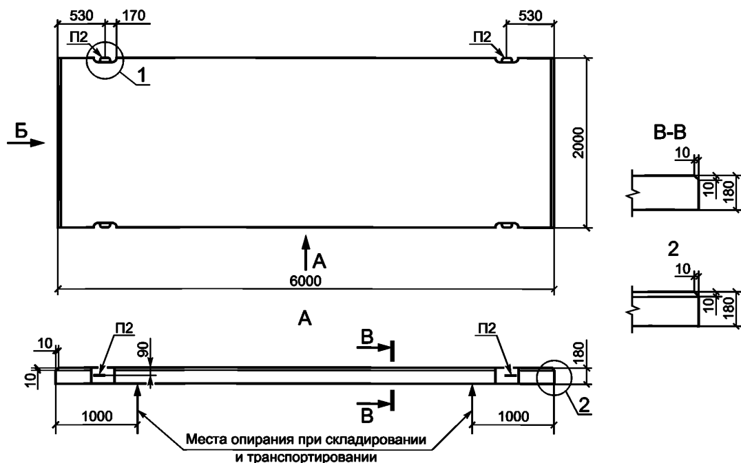
Рисунок 6 — Плита дорожная 2ПДН-18. Общий вид
