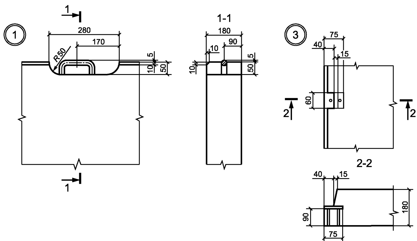
Рисунок 5 — Плита дорожная 1ПДН-18. Узлы 1, 3
