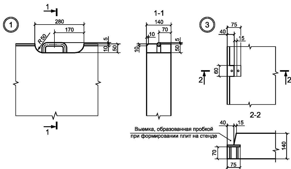
Рисунок 2 — Плита дорожная 1ПДН-14. Узлы 1, 3
