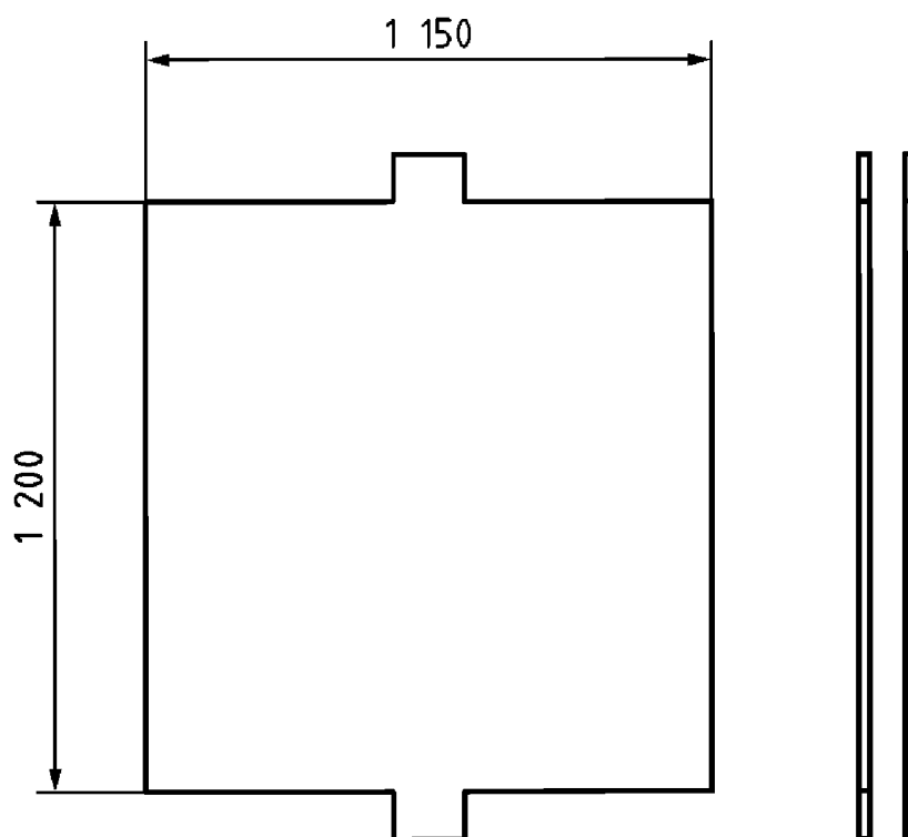
Рисунок D.2 – Эскиз разобранной емкости для проб
