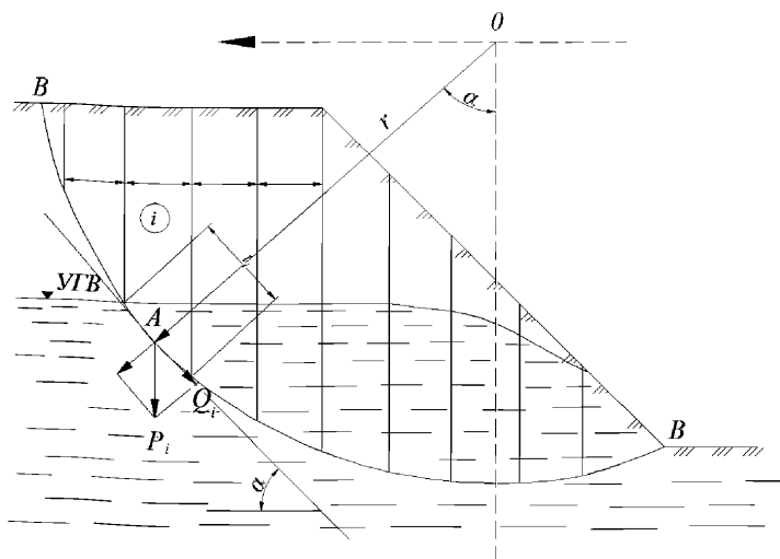
Рисунок 6 – Схема оползневого массива для метода моментов
