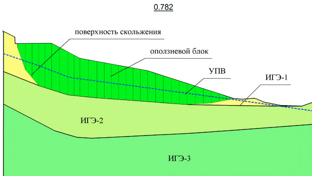
Рисунок Б.5 – Призма обрушения при потере устойчивости склона ( k_{st}=0,782 ).
