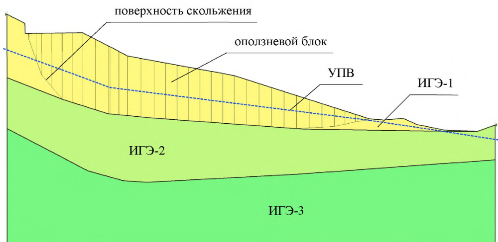
Рисунок Б.1 – Схема к расчету устойчивости склона динамическим методом
