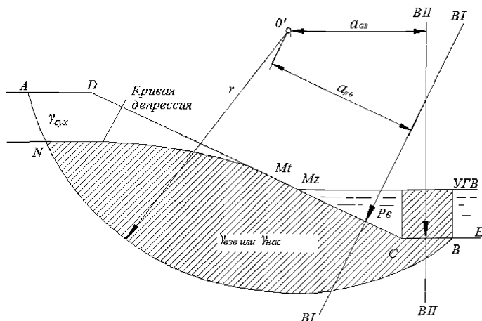
Рисунок 9 – Расчетная схема оползневого склона насыщенного водой
