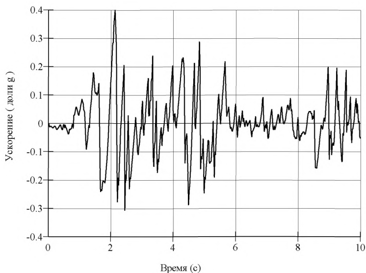
Рисунок Б.2 – Акселерограмма, использованная при динамическом расчете
