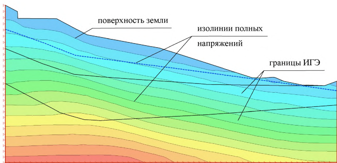
Рисунок Б.3 – Эпюра максимальных полных напряжений в грунтовом массиве при статическом расчете
