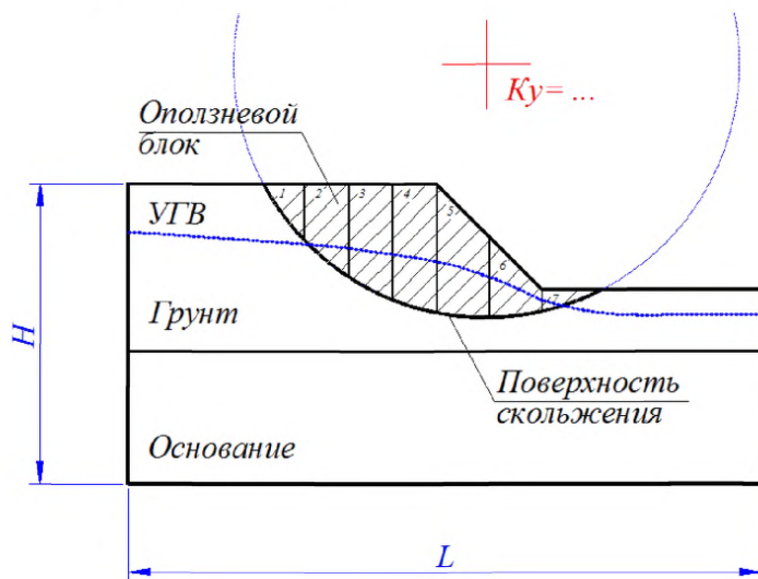
Рисунок 4 – Разбивка оползневого блока на отсеки
