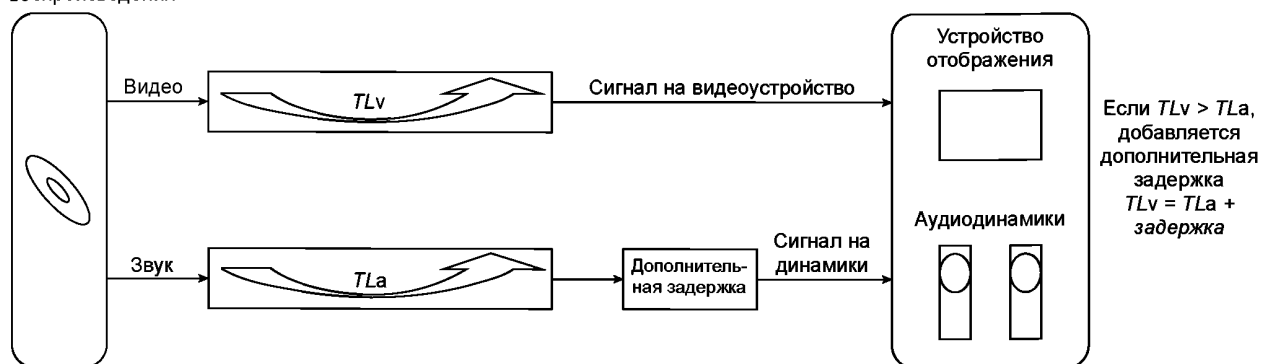
Рисунок Т.2 — Компенсация рассогласования изображения и звука
