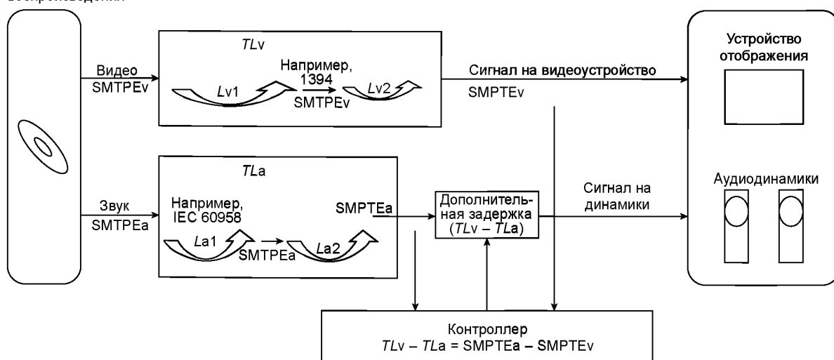
Рисунок Т.3 — Метод передачи временного кода
