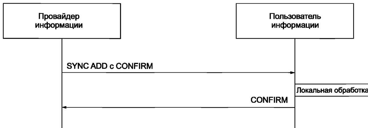
Рисунок A.6 — Транзакция SYNC ADD с подтверждением
