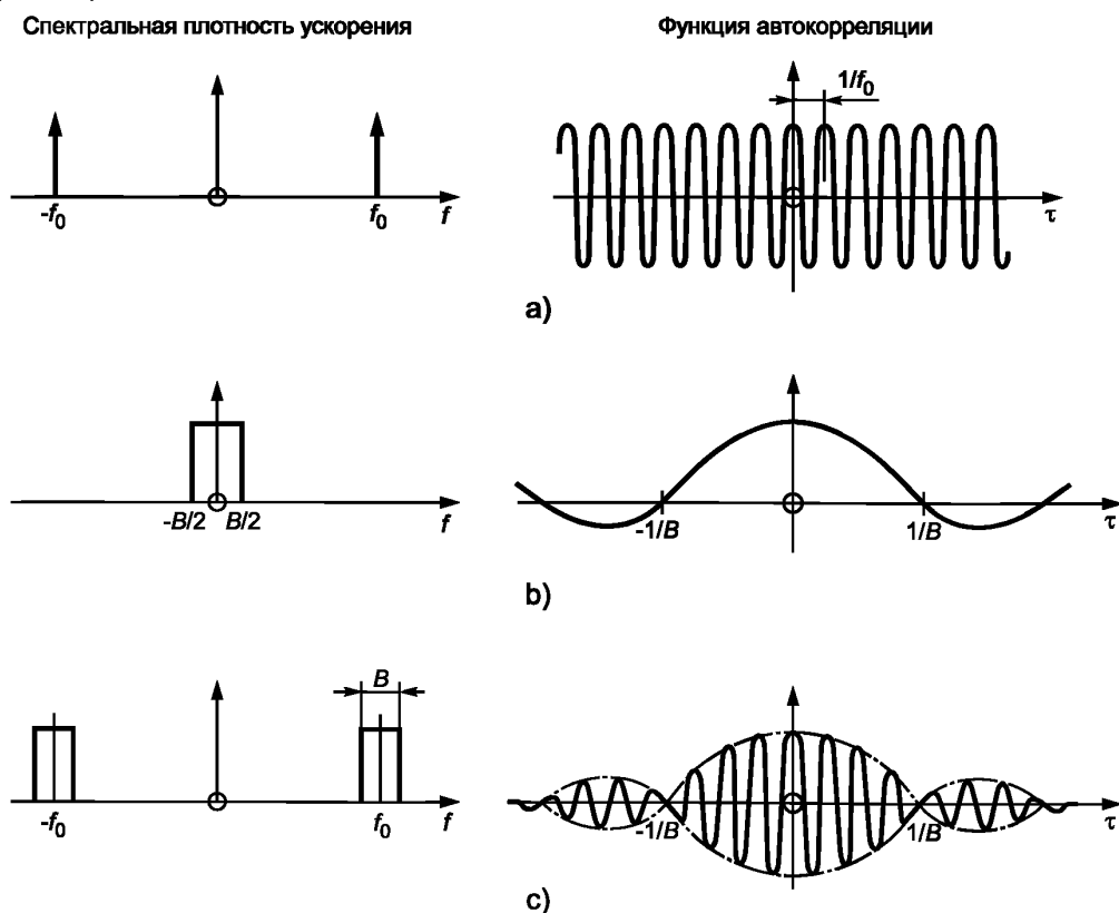
Рисунок 3 — Функции автокорреляции разных сигналов 1)
