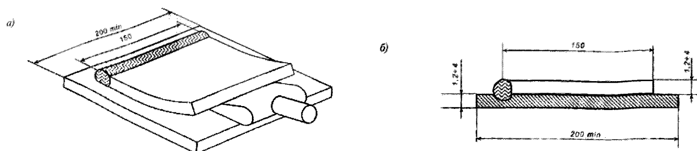
Рис. 3.4 Нахлесточная проба, испытываемая на разъединение пластин:
