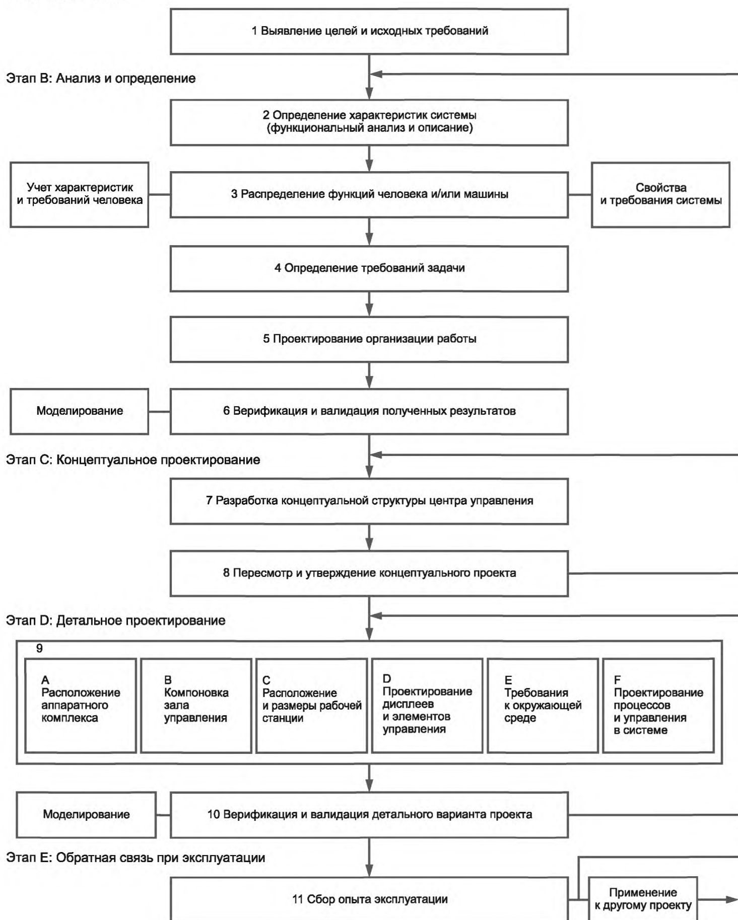
Рисунок 2 — Процесс эргономического проектирования центров управления
