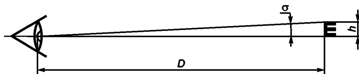
Рисунок А.1 — Параметры, определяющие минимальный угол зрения
