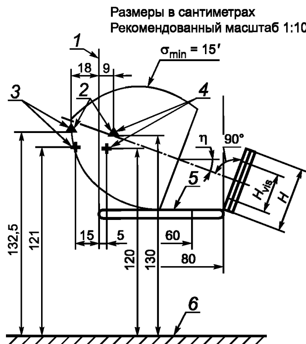
Рисунок А.4 — Схема пространства идентификации (вид сбоку)
