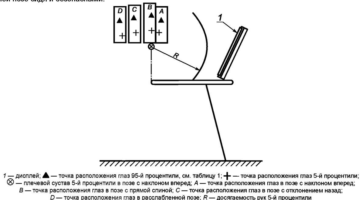
Рисунок 3 — Рабочие позы сидя, соответствующие таблице 1
