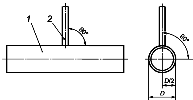
1 — тестируемый ствол; 2 — пучок лазерного излучения
