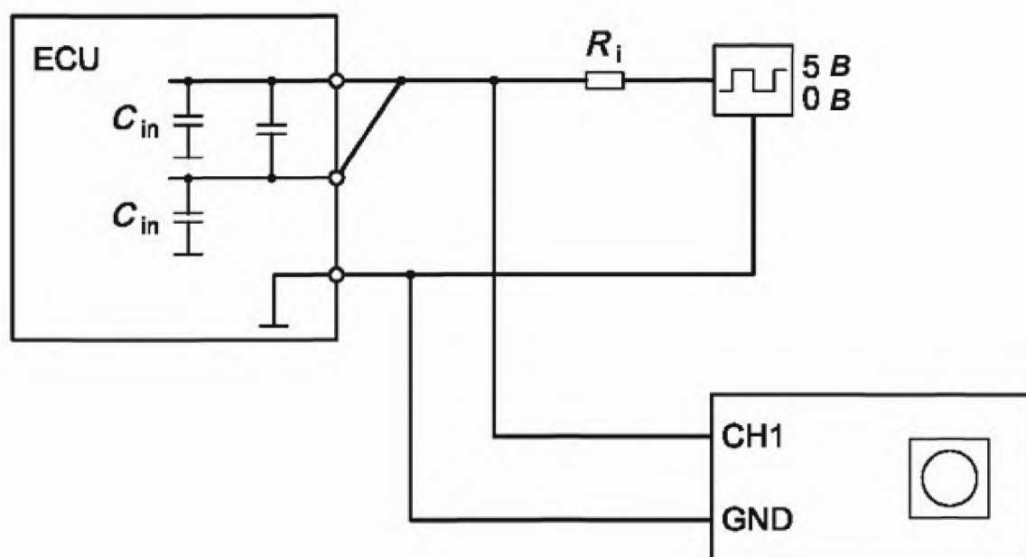
Рисунок 10 — Измерение входной емкости, C_{\text{busin}} , узла CAN в рецессивном состоянии
