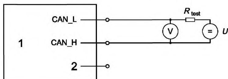
1 — узел CAN со схемой оконечной нагрузки; 2 — заземление
