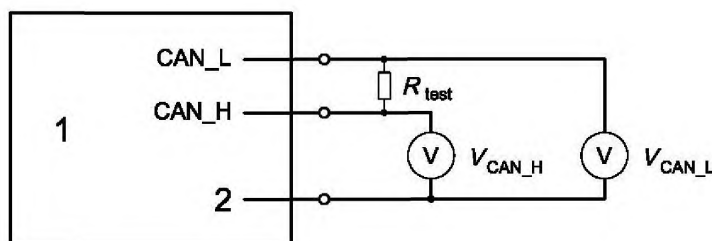
1 — узел CAN со схемой оконечной нагрузки; 2 — заземление
