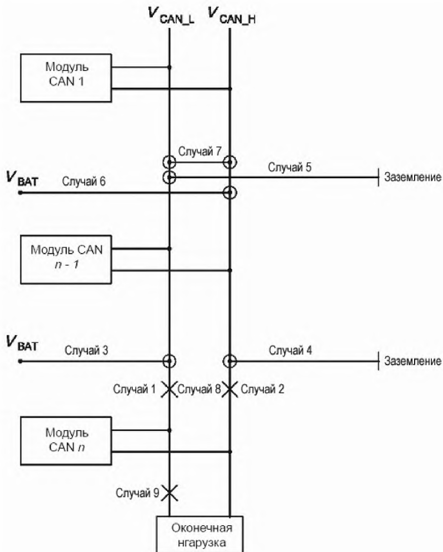
Рисунок 19 — Возможные отказы линий шины
