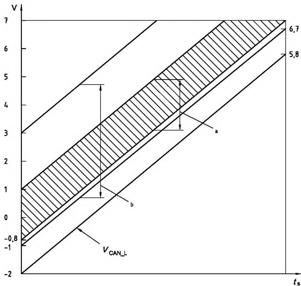
t_s — случайное время; a — реальный диапазон значений V_{CAN\_H} на линии шины; b — диапазон V_{CAN\_H} для приема
