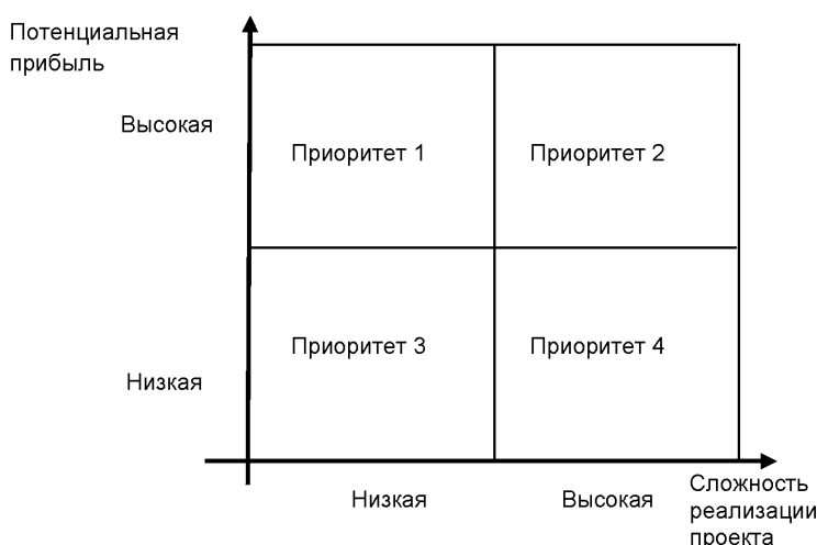
Рисунок 5 — Схема ранжирования
