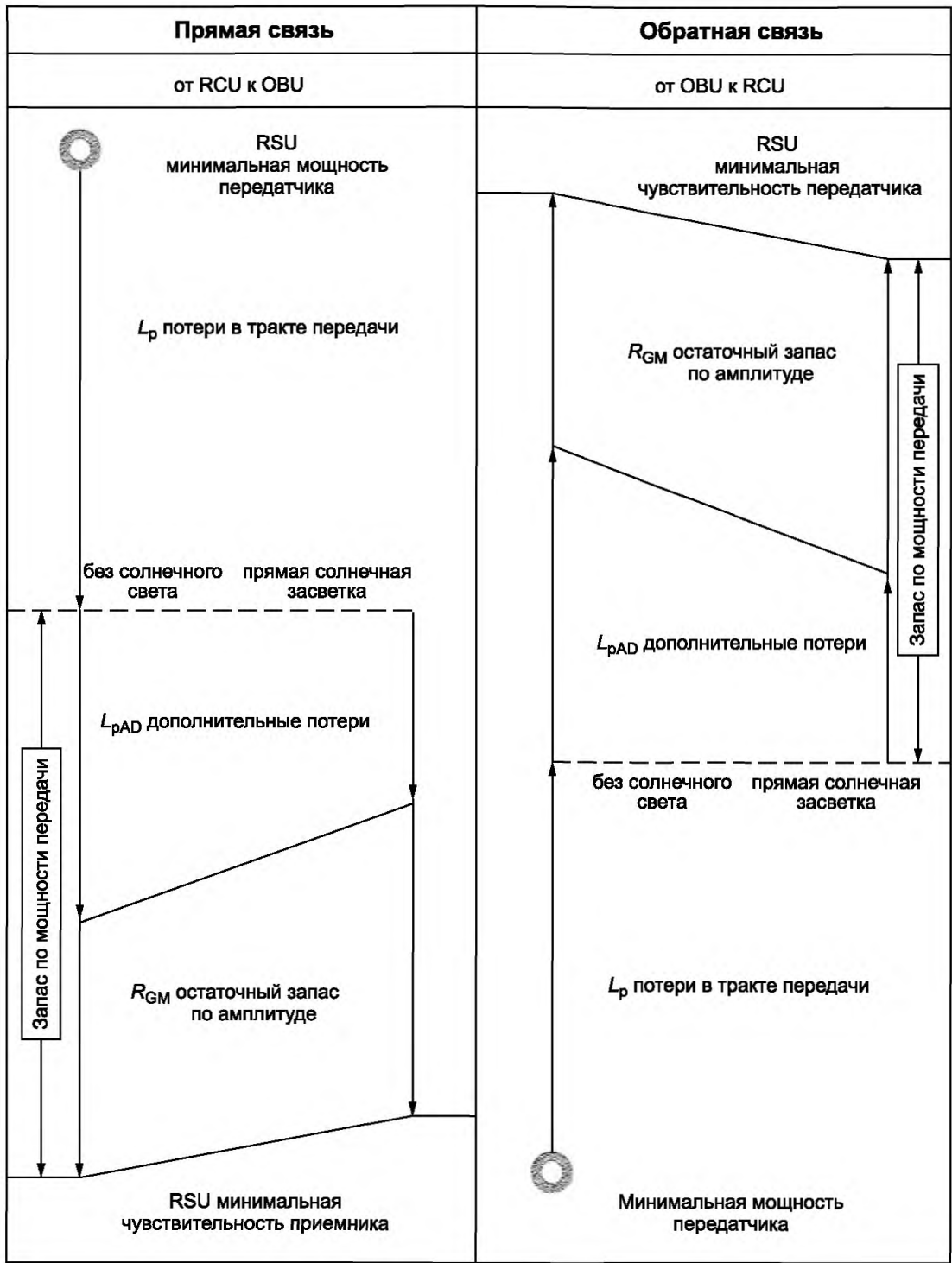
Рисунок С.1 — Схема бюджета питания связи
