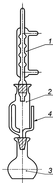
1 — холодильник; 2 — экстрактор; 3 — экстракционная колба; 4 — сифонная трубка
