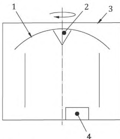
1 — подвижный купол; 2 — вакуумная камера; 3 — распылитель; 4 — испаритель покрытия
