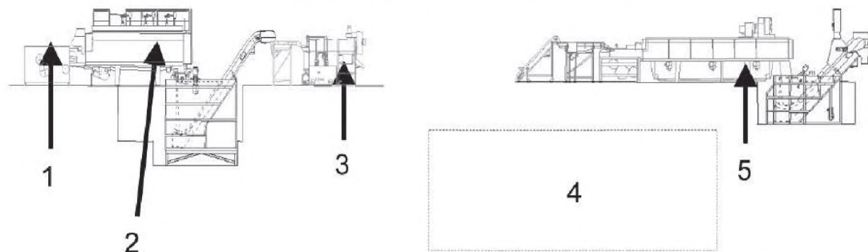
1 — погрузка; 2 — конвейерная печь для термообработки деталей; 3 — машина для промывки снизу или промывной бак; 4 — некоторые процессы (например, изотермическая закалка), не использующие печь; 5 — термообработка деталей в печи
