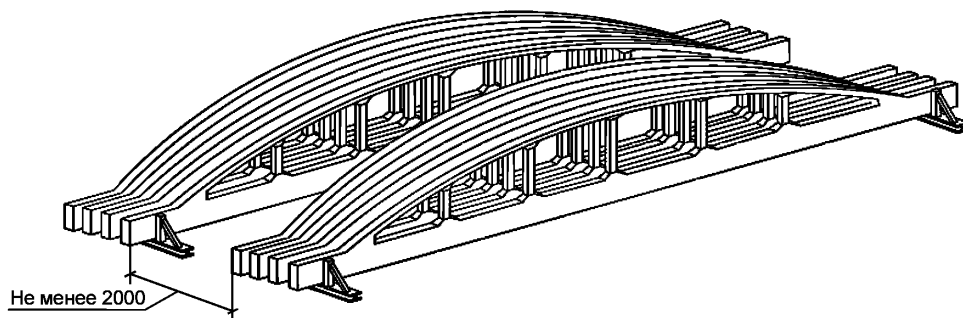
Рисунок 1 — Складирование ферм
