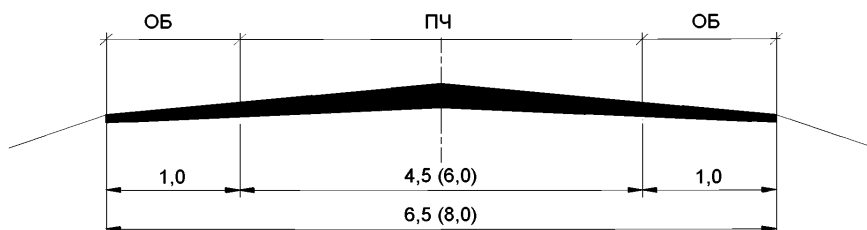
д) Поперечные профили подъездных автомобильных дорог VB категорий для подъездов к сельскохозяйственным угодьям, где ПЧ – проезжая часть, КП – краевая полоса у обочины, ОБ - обочина, УО – укрепленная часть обочины, ГО - ширина грунтовой части обочины. Размеры геометрических элементов даны в метрах.
