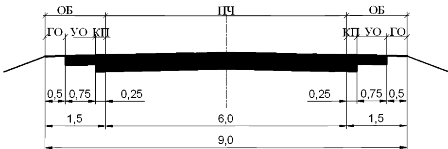
б) Поперечные профили распределительных автомобильных дорог IVБ-р категории и подъездов IVА-п и IVБ-п, категорий
