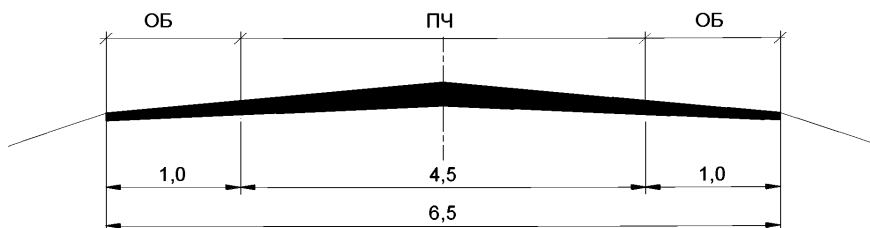
г) Поперечные профили подъездных автомобильных дорог VB категорий (подъезды к промышленным предприятиям и месторождения полезных ископаемых, кроме подъездов к сельскохозяйственным угодьям)
